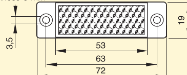
CTR10-RFL000018 Spessore 9,5 mm Thickness 9,5 mm
