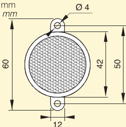
CTR1-RFL000012 ADESIVO Spessore 6 mm Thickness 6 mm
